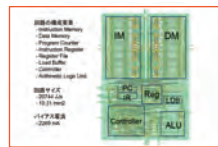
超伝導体デバイスを用いたマイクロプロセッサの設計
