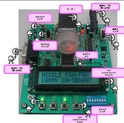
図 :組み込み系プログラミング教材
